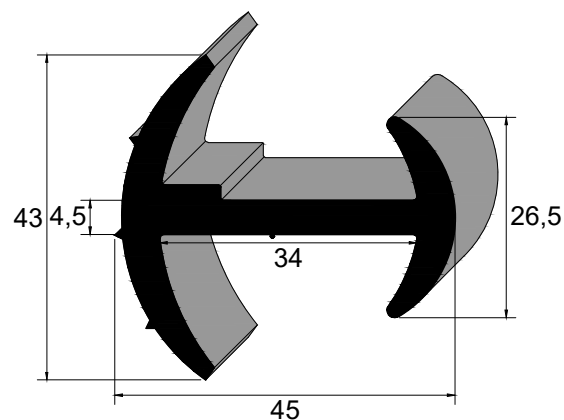
IBC 3038 SBR 80 Sh A Vedação Porta Furgões
