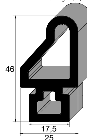
IBC 3295 EPDM 80 Sh A Vedação Porta de Secadora de Madeira
