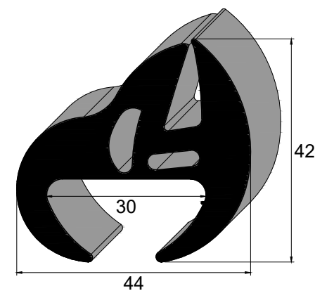
IBC 8061 EPDM 60 Sh A
