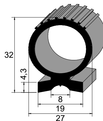
IBC 3135 EPDM 65 Sh A Vedação Porta de Secadora de Madeira
