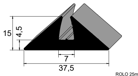
IBC 3492 NBR 80 Sh A Vedação Forma de Pré-Moldados
