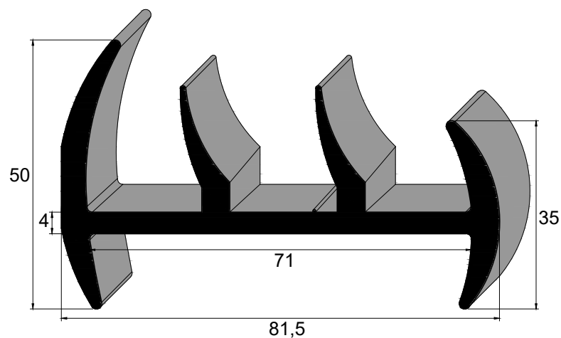
IBC 3763 SBR 75 Sh A Vedação Furgões Frigoríficos
