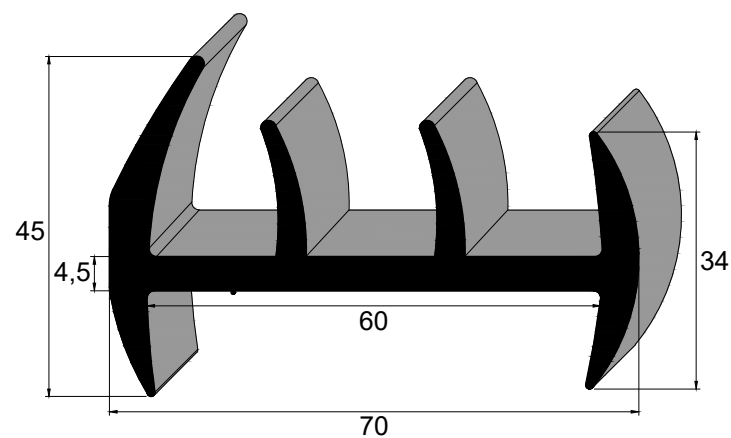
IBC 3693 EPDM 70 Sh A Vedação Porta Frigorífico
