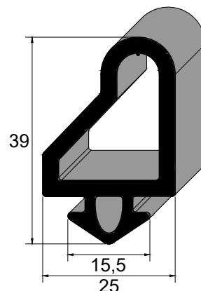
IBC 3135 EPDM 65 Sh A Vedação Porta de Secadora de Madeira
