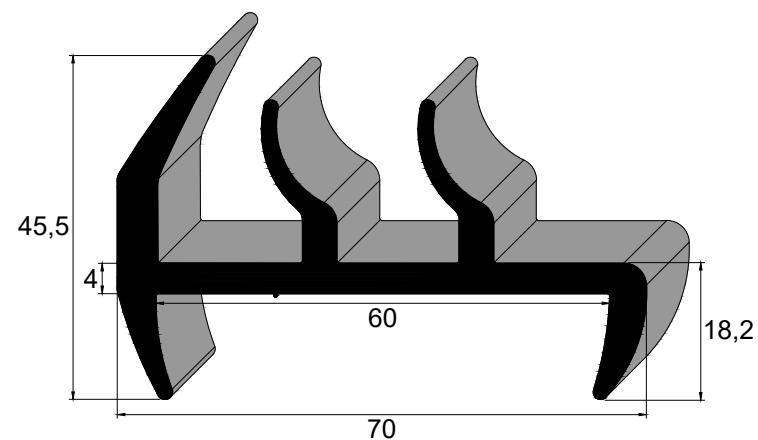
IBC 3538 EPDM 75 Sh A Vedação Porta Frigorífico
