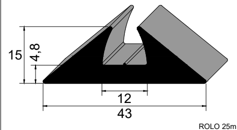
IBC 3526 NBR 75 Sh A Vedação Forma de Pré-Moldados
