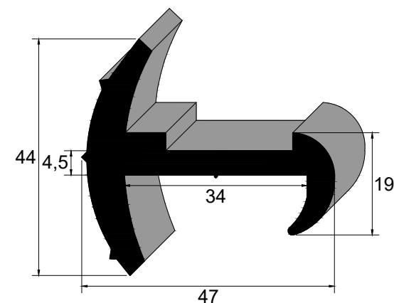
IBC 3436 SBR 75 Sh A Vedação Porta Furgões
