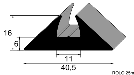
IBC 3548 NBR 80 Sh A Vedação Forma de Pré-Moldados
