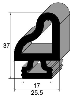
IBC 3320 SBR 80 Sh A IBC 7129 SBR 80 Sh A Vedação Porta Ônibus Comil Svelto I, Svelto II, Doppio Versatile
