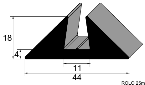
IBC 3701 NBR 75 Sh A Vedação Forma de Pré-Moldados
