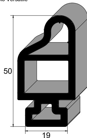
IBC 3320 SBR 80 Sh A IBC 7129 SBR 80 Sh A Vedação Porta Ônibus Comil Svelto I, Svelto II, Doppio Versatile
