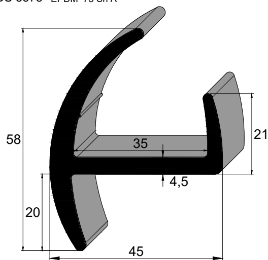
IBC 3578 EPDM 75 Sh A
