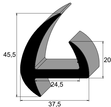
IBC 3409 SBR 80 Sh A Vedação Porta Container
