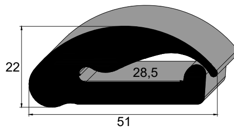
IBC 8032 SBR 60 Sh A Aro de Roda Ônibus Caio, Metalbus e Thanco
