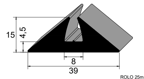
IBC 3488 NBR 80 Sh A Vedação Forma de Pré-Moldados
