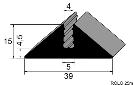
IBC 3605 NBR 80 Sh A Vedação Forma de Pré-Moldados
