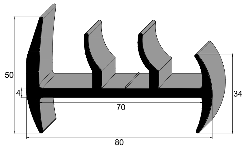
IBC 3768 SBR 75 Sh A Vedação Furgões Frigoríficos Randon
