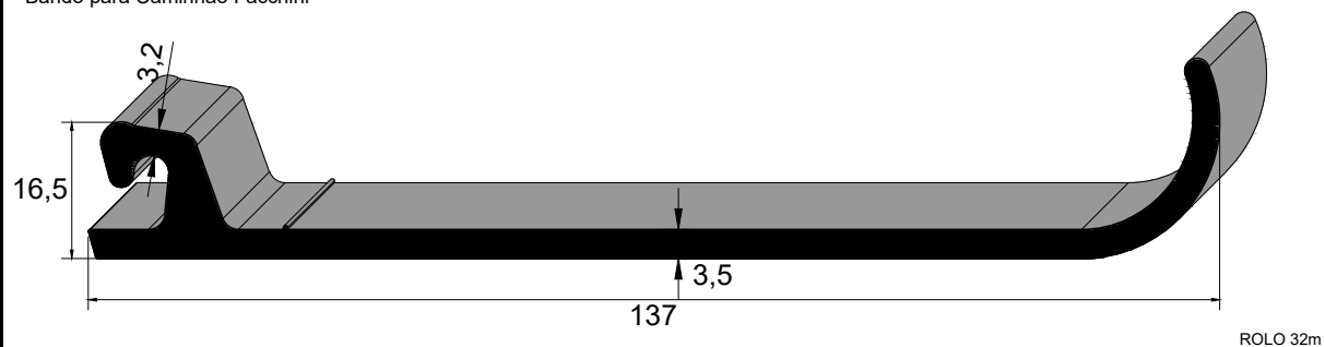
IBC 3799 EPDM 75 Sh A Bandô para Caminhão Facchini
