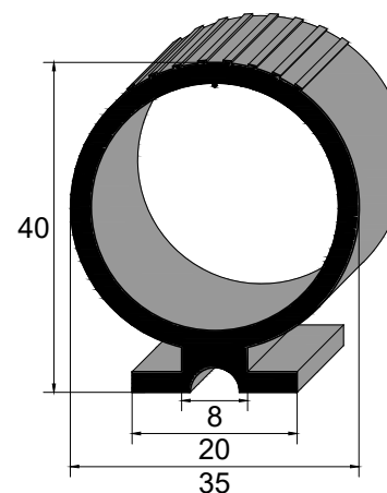
IBC 3295 EPDM 80 Sh A Vedação Porta de Secadora de Madeira
