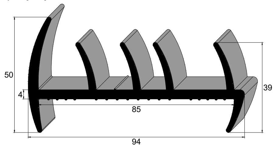
IBC 3806 EPDM 75 Sh A Vedação Furgão Frigorífico
