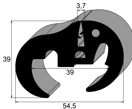
IBC 8051 SBR 60 Sh A Vedação Cabine Máquina Agrícola
