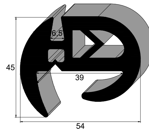
IBC 8039 EPDM 60 Sh A Janela Lateral Ônibus Comil
