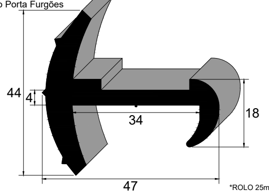
IBC 3661 SBR 80 Sh A Vedação Porta Furgões
