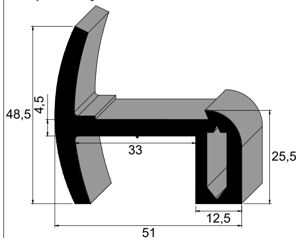
IBC 3785 EPDM 80 Sh A Vedação Porta Furgão
