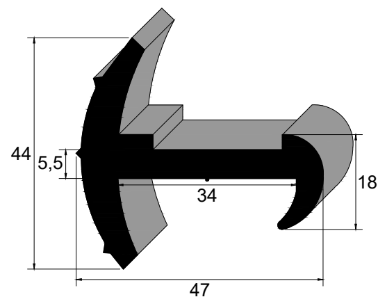
IBC 3038 SBR 80 Sh A Vedação Porta Furgões
