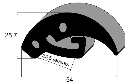
IBC 8065 SBR 60 Sh A Aro de Roda Ônibus MP Rodoviário/ Torino GIV
