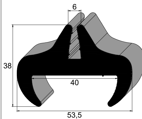
IBC 8048 SBR 60 Sh A Vedação Cabine Máquina Agrícola/ Ônibus
