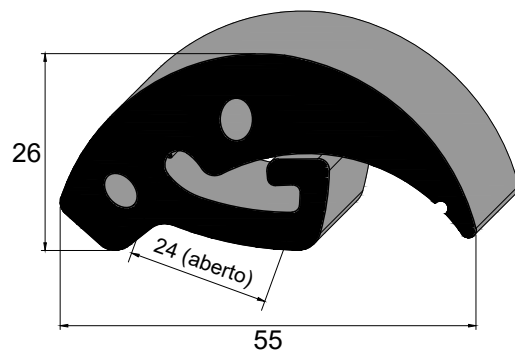
IBC 8066 SBR 60 Sh A Aro de Roda Ônibus Ciferal Padron, MP Rodoviário GIV/ Torino GIV e GV
