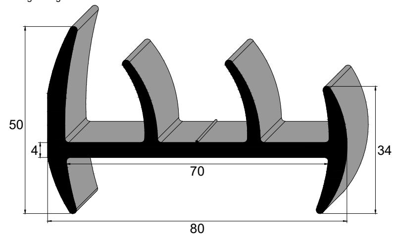
IBC 3795 SBR 75 Sh A Vedação Furgão Frigorífico
