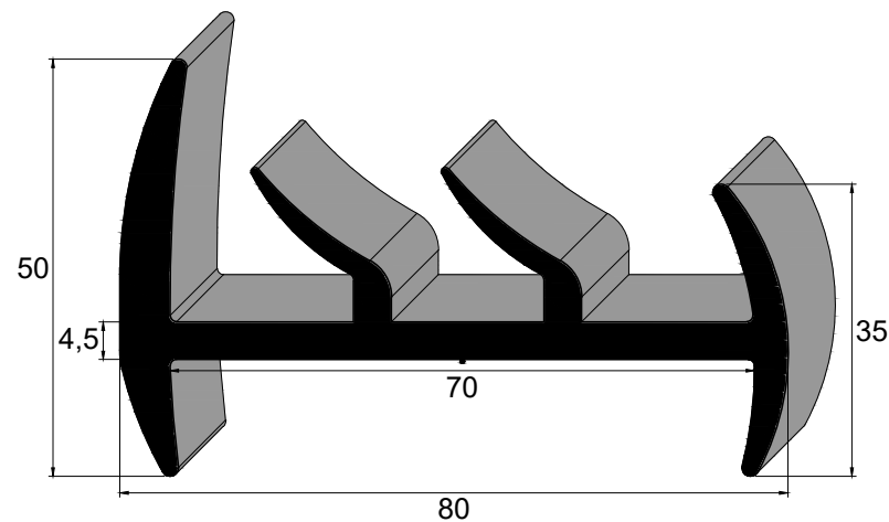
IBC 3768 SBR 75 Sh A Vedação Furgões Frigoríficos Randon
