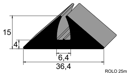
IBC 3697 NBR 80 Sh A Vedação Forma de Pré-Moldados
