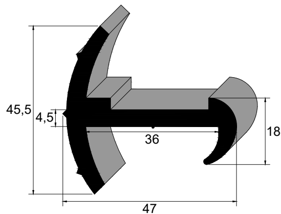
IBC 3661 SBR 80 Sh A Vedação Porta Furgões
