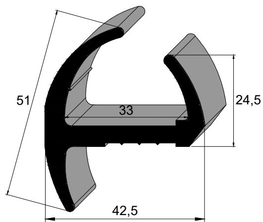
IBC 3279 SBR 80 Sh A Vedação Porta Container
