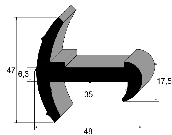
IBC 3436 SBR 75 Sh A Vedação Porta Furgões
