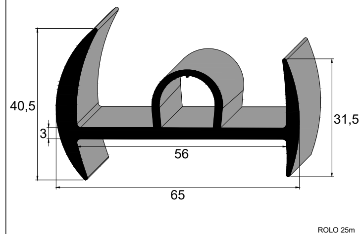
IBC 3509 EPDM 70 Sh A Vedação Porta Furgão Carropel
