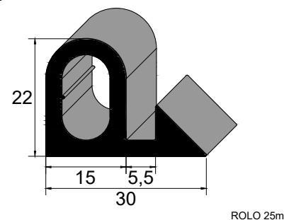
IBC 3529 NBR 75 Sh A Vedação Forma de Pré-Moldados
