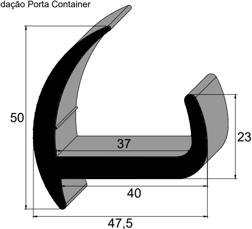
IBC 3205 SBR 80 Sh A IBC 3451 EPDM 80 Sh A Vedação Porta Container
