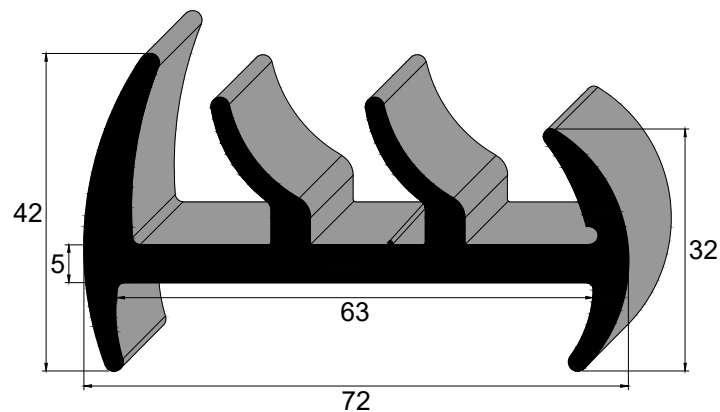
IBC 3693 EPDM 70 Sh A Vedação Porta Frigorífico
