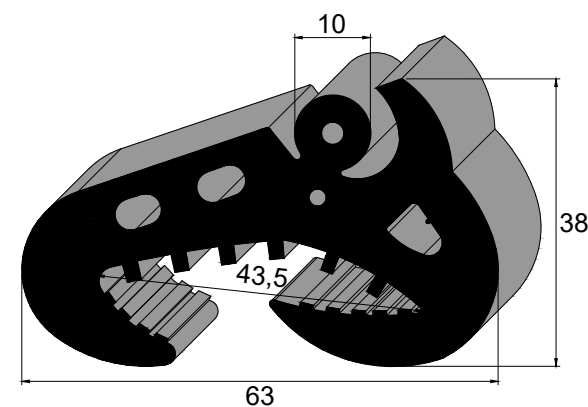
IBC 8039 EPDM 60 Sh A Janela Lateral Ônibus Comil
