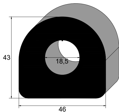
IBC 3207 SBR 80 Sh A
