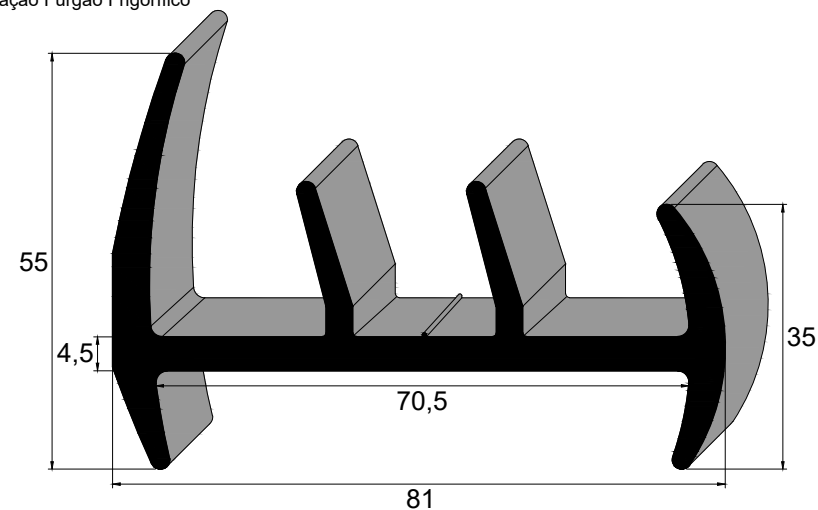
IBC 3806 EPDM 75 Sh A Vedação Furgão Frigorífico
