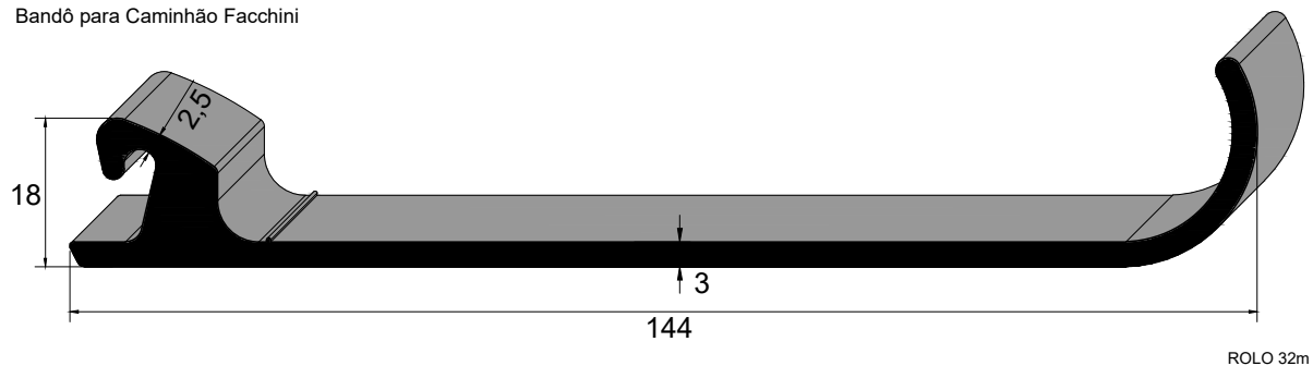
IBC 3766 SBR 75 Sh A Bandô para Caminhão Facchini
