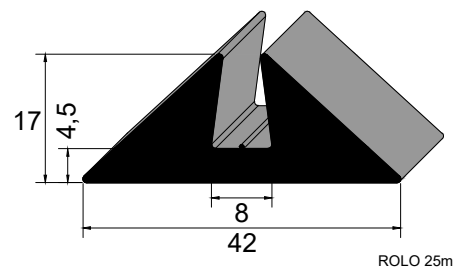
IBC 3529 NBR 75 Sh A Vedação Forma de Pré-Moldados
