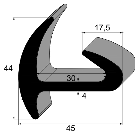
IBC 3241 SBR 80 Sh A Vedação Porta Container
